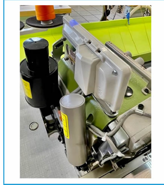
DISPOSITIVI ELETTROMAGNETICI PER S851 E ALZAPIEDINO ELECTRONIC DEVICE FOR S851 AND FOOT LIFTER
