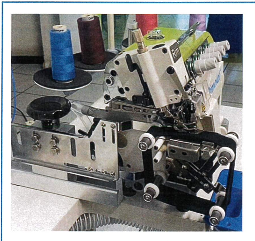
TENSIONATORE ELASTICO RTP ELASTIC TENSIONER RTP
