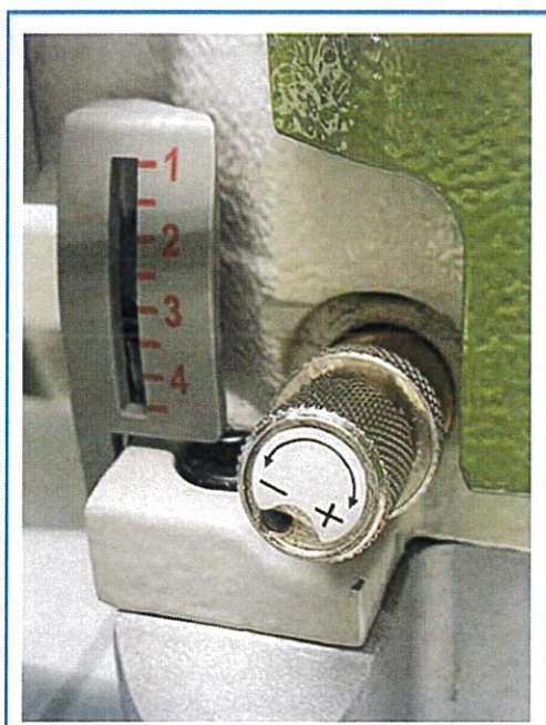
ALLUNGAPUNTO/STITCH REG.
