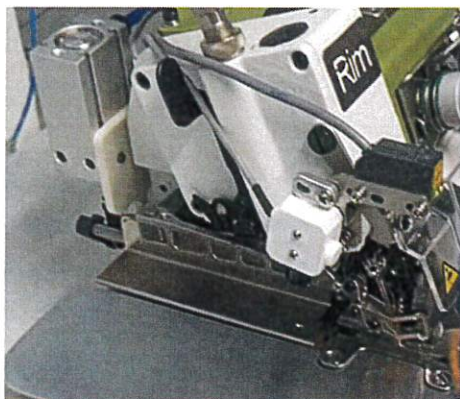
TAGLIACATENELLA CHAIN CUTTER
