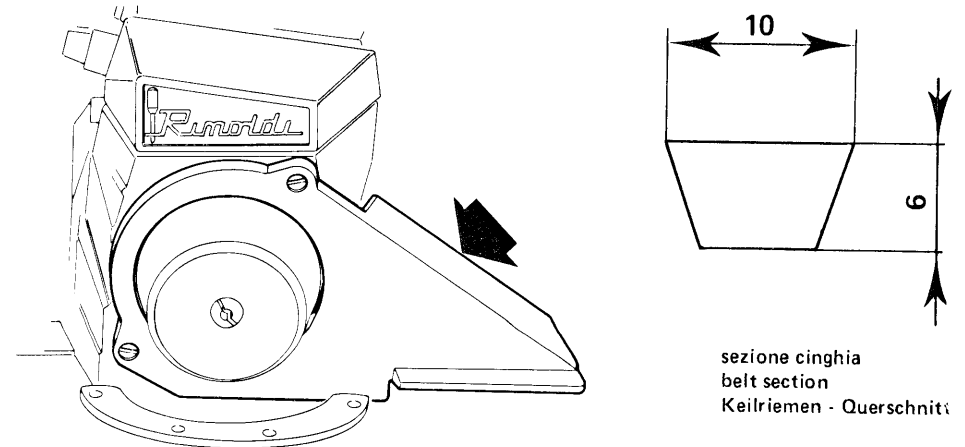
coperchio protezione cinghia belt guard cover Riemen-Schutzdeckel
